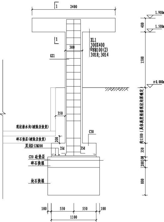
图 1.3 2.4m 宽混凝土管架立面图
