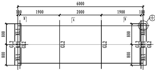
图 1.10 1.6m 宽混凝土管架平面图
