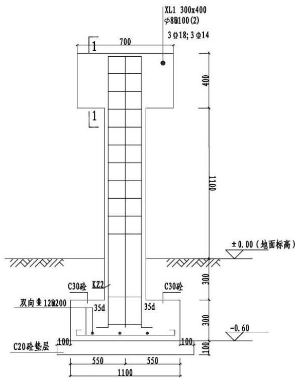
图 1.13 0.7m 宽混凝土管架立面图
