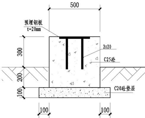
图 1.15 0.5m 宽混凝土支墩剖面图
