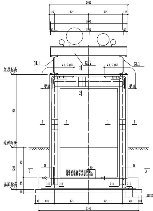
图 1.9 2.0m 宽双柱混凝土管架立面图
