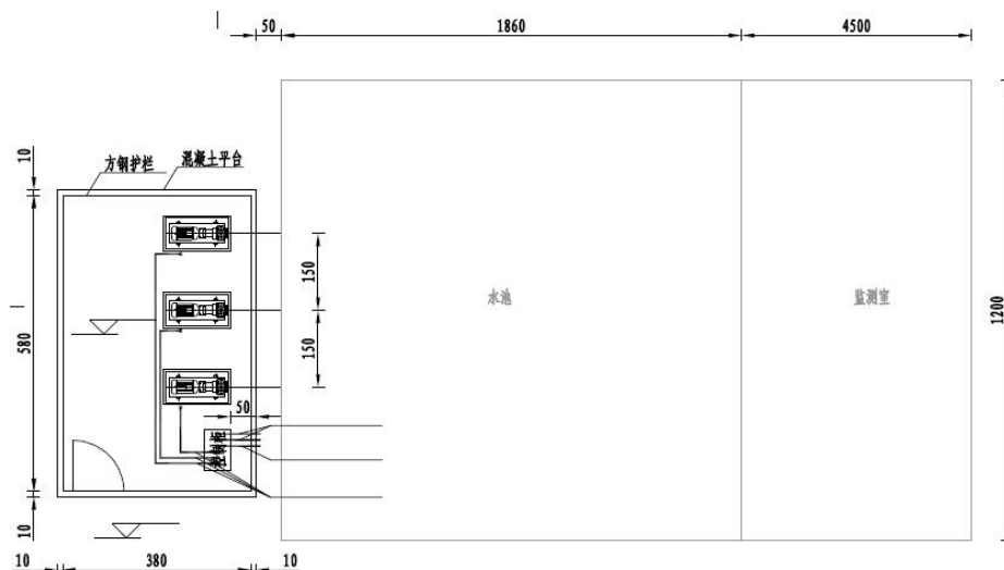
图 1.18 水泵安装平面示意图
