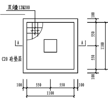
图 1.2 2.4m 宽混凝土管架基础平面图
