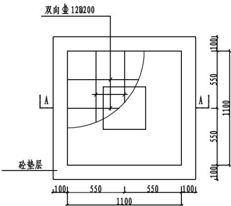
图 1.14 0.7m 宽混凝土管架基础平面图
