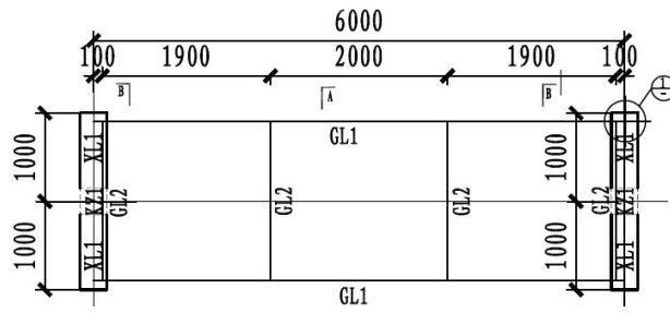
图 1.7 2.0m 宽双柱混凝土管架平面示意图
