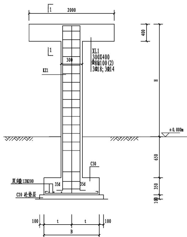
图 1.6 2.0m 宽混凝土管架立面图
