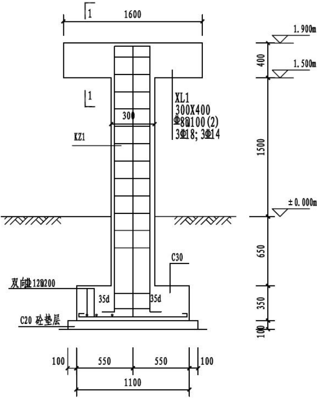
图 1.12 1.6m 宽混凝土管架立面图
