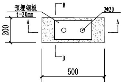
图 1.16 0.5m 宽混凝土支墩平面图
