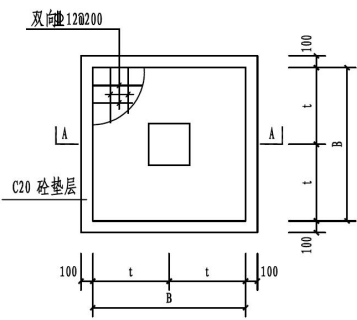
图 1.5 2.0m 宽混凝土管架基础平面图
