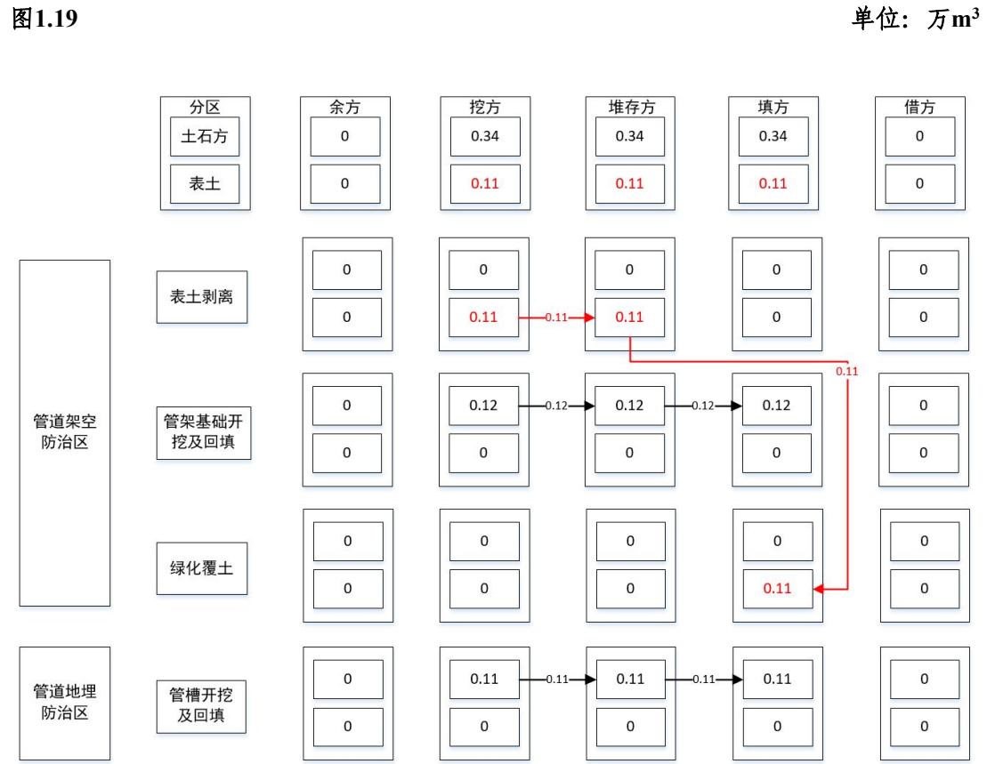
土石方流向框图
