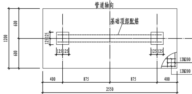
图 1.8 2.0m 宽双柱混凝土管架基础平面示意图
