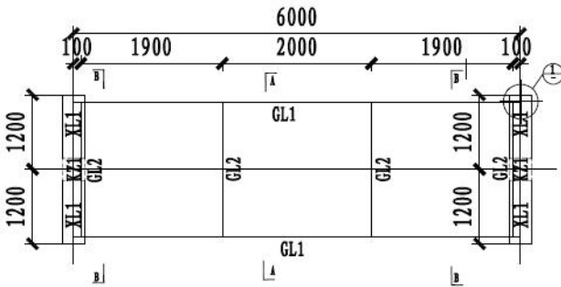
图 1.1 2.4m 宽混凝土管架平面示意图
