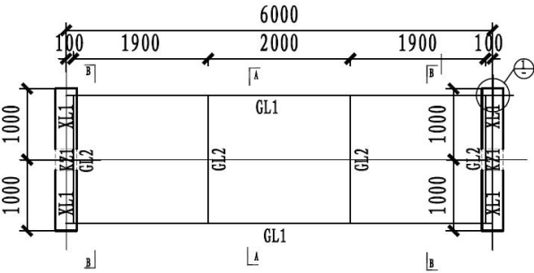
图 1.4 2.0m 宽混凝土管架平面示意图
