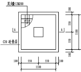
图 1.11 1.6m 宽混凝土管架基础平面图
